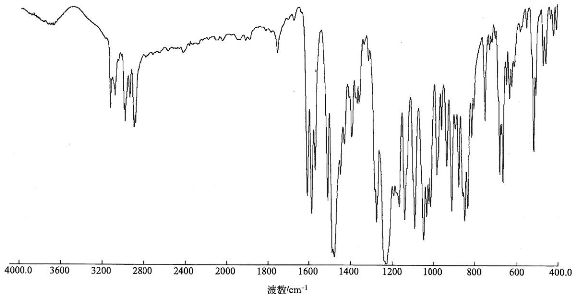
图 1 苯醚甲环唑标样的红外光谱图
